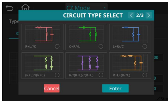
图 6：多模式负载仿真
