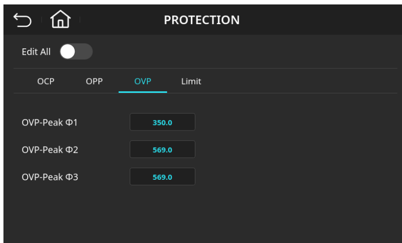
图 4-56 输出过电压保护页面(OVP-Peak \Phi 1 = 350\text{ V} )
