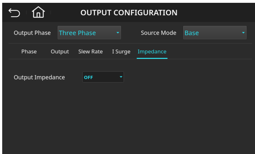
图 4-46 可程序设计输出阻抗功能（Impedance）页面
