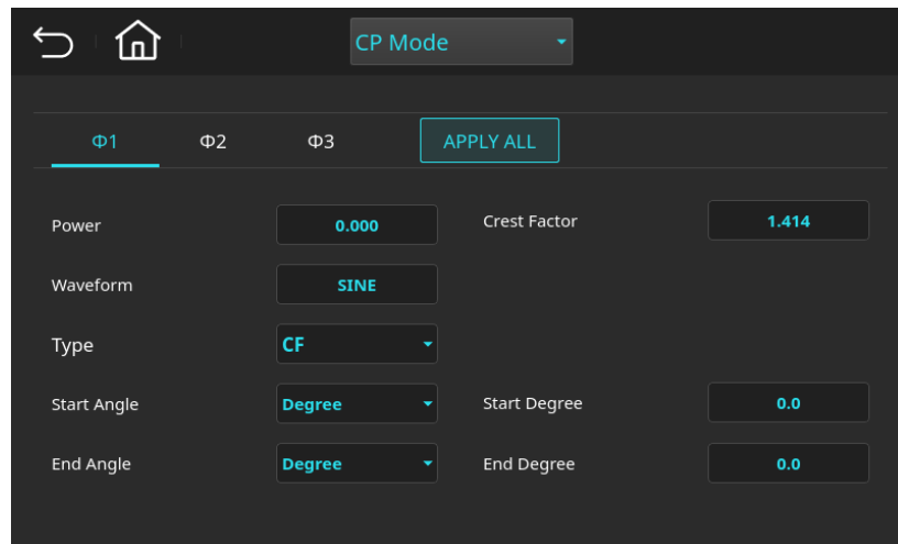
图 9-3 定功率操作模式(CP Mode)页面
