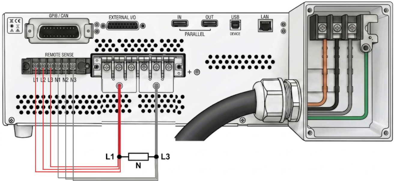
图 3-7 单相模式输出和远程量测线接线方式
