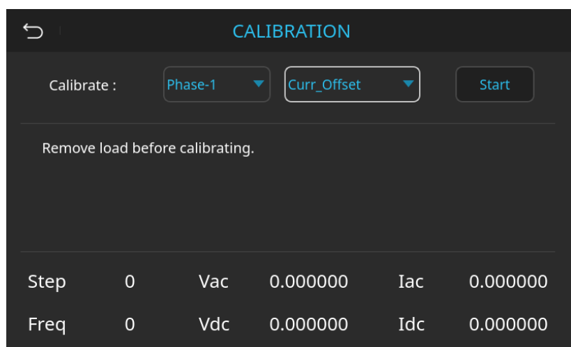
图 8-18 校准输出偏移电程序
