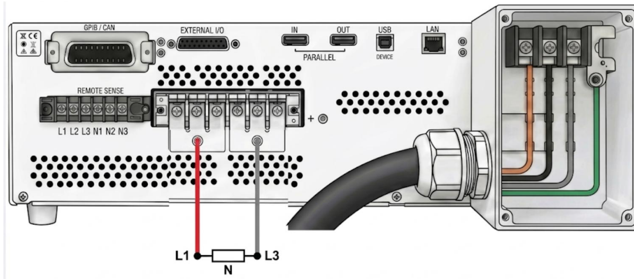
图 3-4 输出单相模式接线方式
