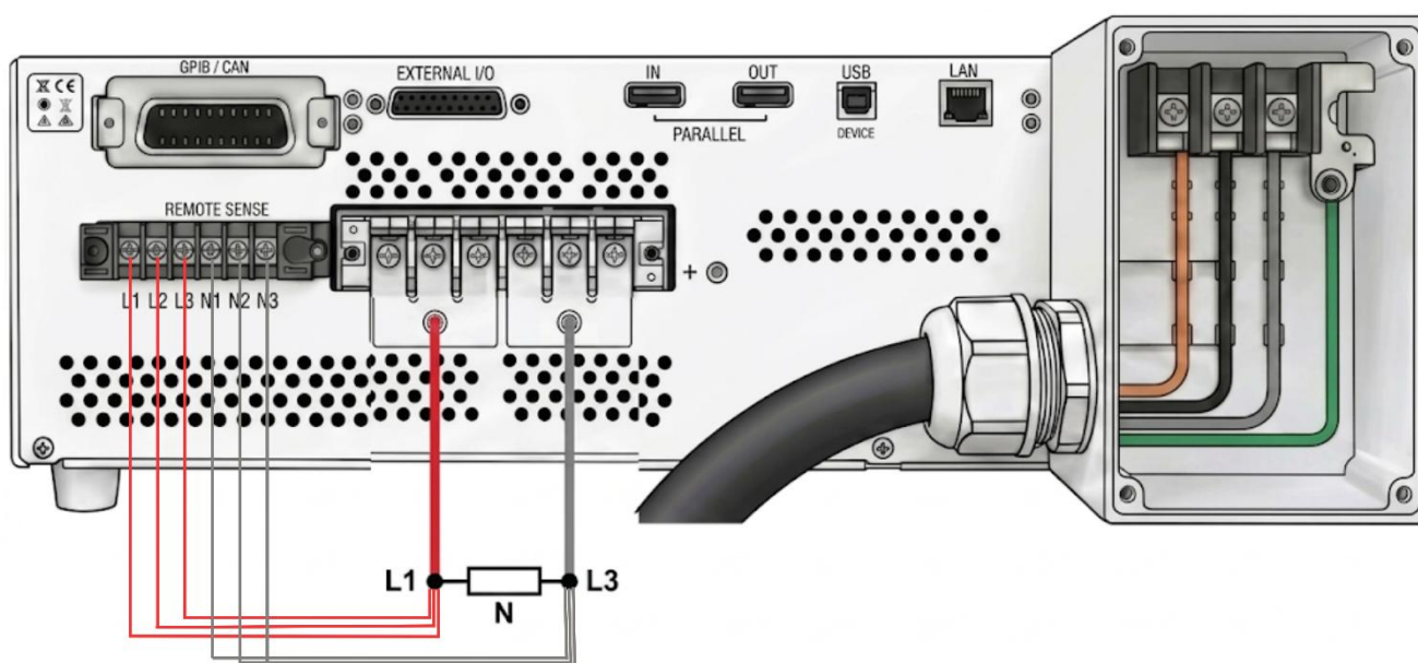
图 3-7 单相模式输出和远程量测线接线方式
