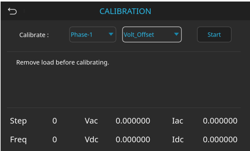
图 8-5 校准第一相的输出偏移电压画面
