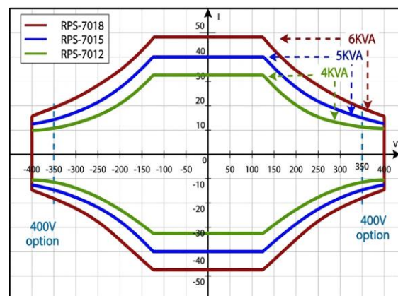
图 1-2 直流电压/电流操作范围图-单相模式
