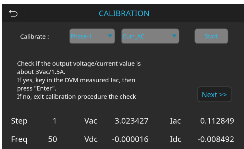
图 8-22 校准输出交流电程序-输出 3Vac
