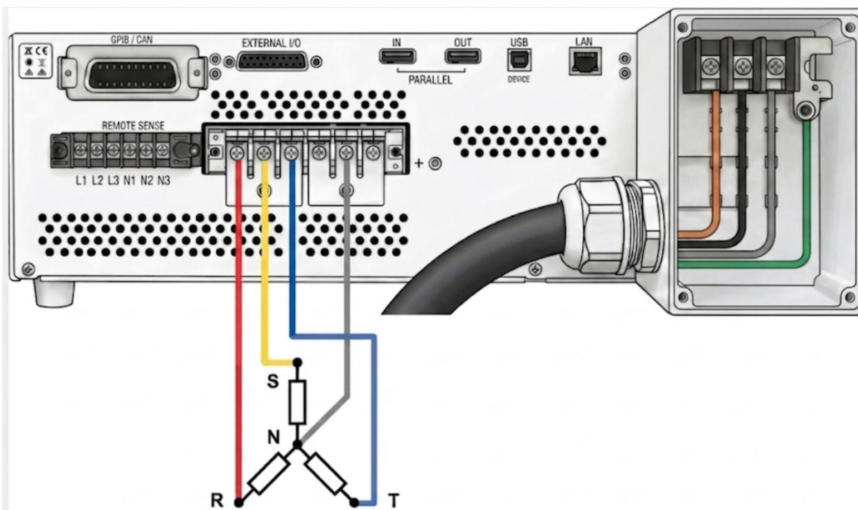
图 3-3 输出三相模式接线方式
