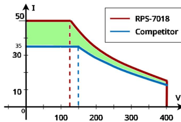
图 1-1 交流电压/电流操作范围图-三相模式
